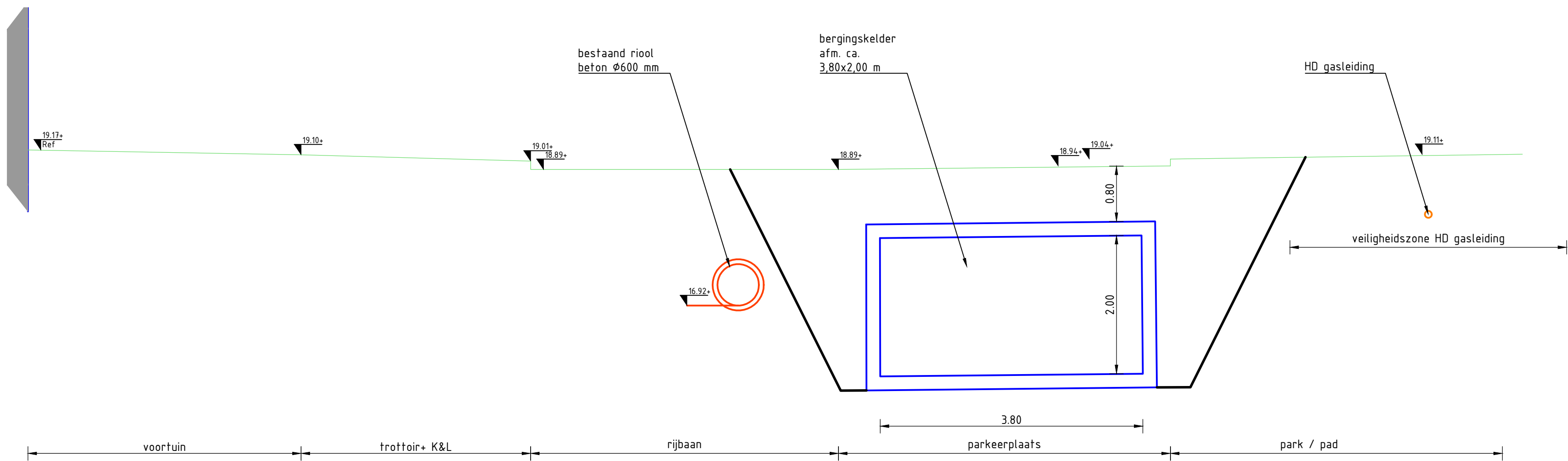
Principe dwarsprofiel A-A schaal 1:50
